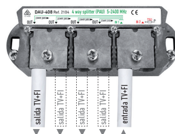
Conexión para una instalación DAU modo distribuidor
