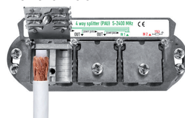
Insertión del vivo del cable en el orificio
