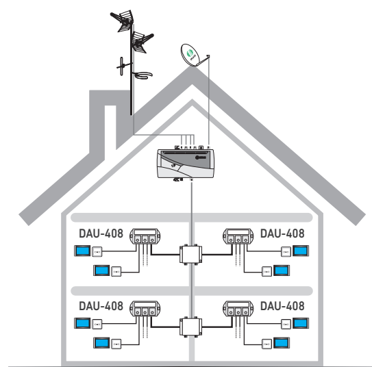
Ejemplo de aplicación (modo distribuidor)
