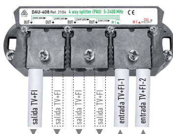
Conexión para una instalación modo DAU+PAU (ICT)
