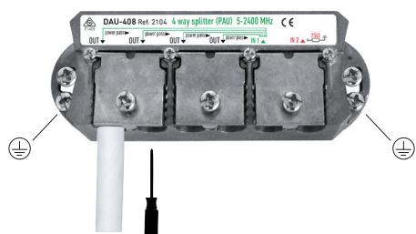
Cierre de la tapa-brid mediante el tornillo
